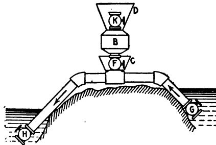
FIG. 21.—Syphon.
